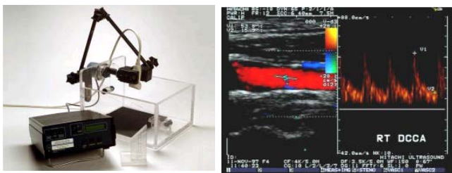
Doppler String Phantom
